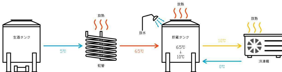
火入れ～貯蔵工程 廃熱回収例
