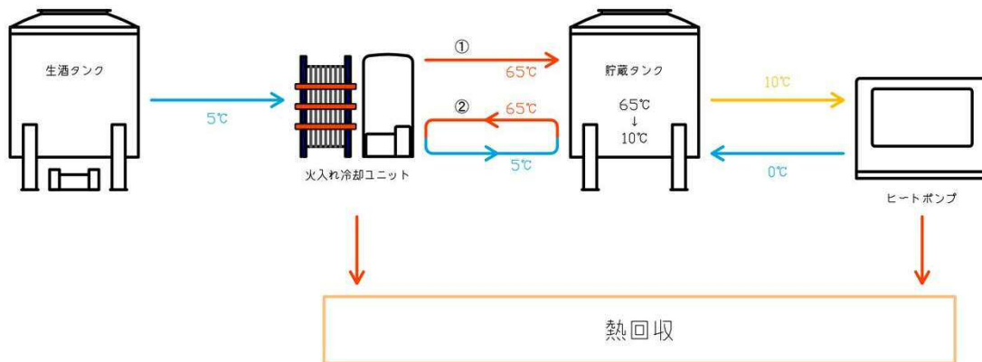
火入れ～貯蔵工程 廃熱回収例
